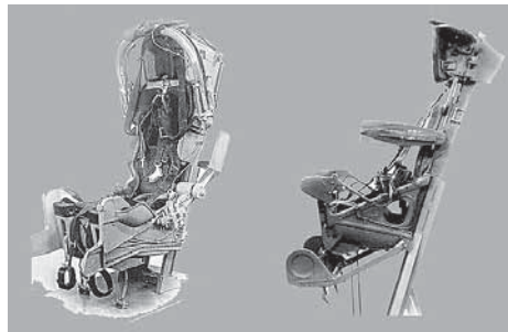
Катапультное кресло К-1
